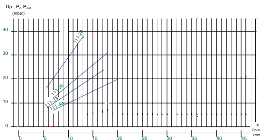
ABAQUES DE PERTES DE CHARGE
